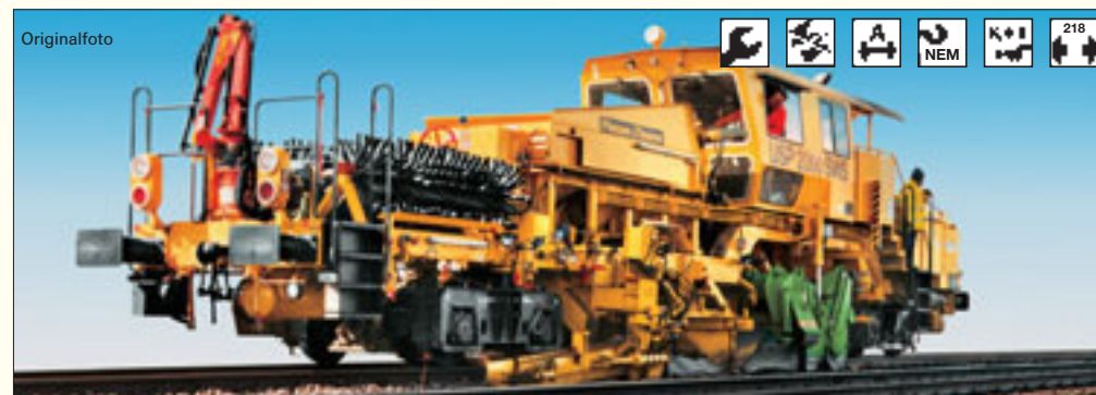
B-16060 Schotterverteil- und Profiliermaschine USP 2000 SWS
